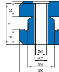
Abb. 5 MO-Lager Typ III
