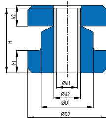
Abb. 4 MO-Lager Typ II
