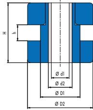
Abb. 3 MO-Lager Typ I
