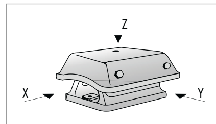
Abb. 2 Hauptbelastungsrichtungen
